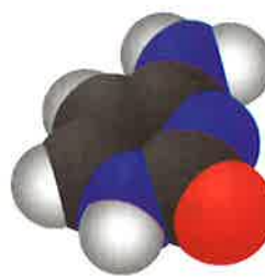
Cytosine
